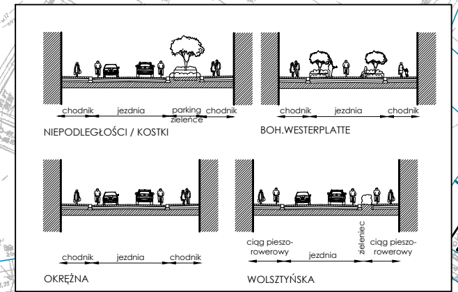
PRZEKROJE CHARAKTERYSTYCZNE ULIC
